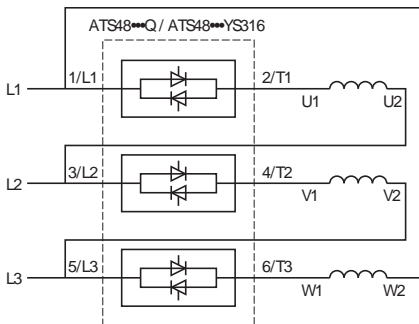
Schaltung in der Dreieckwicklung des Motors (Wurzel-3-Schaltung)
